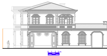
Elevation 02
