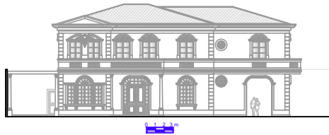
Elevation 01
